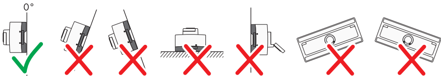
Afbeelding 3: Montagepositie
