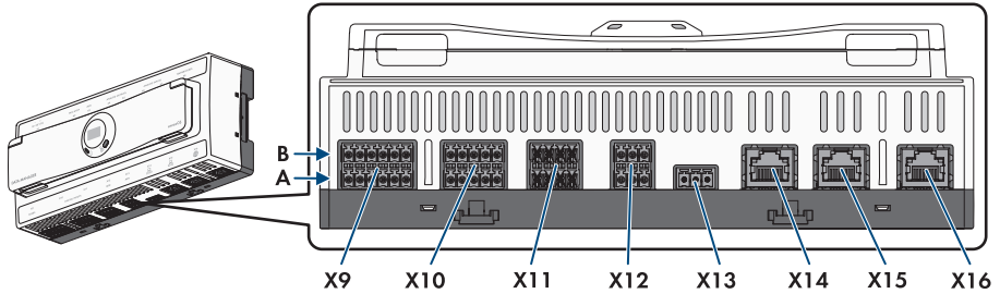
Afbeelding 7: Overzicht van onderste aansluitpaneel
