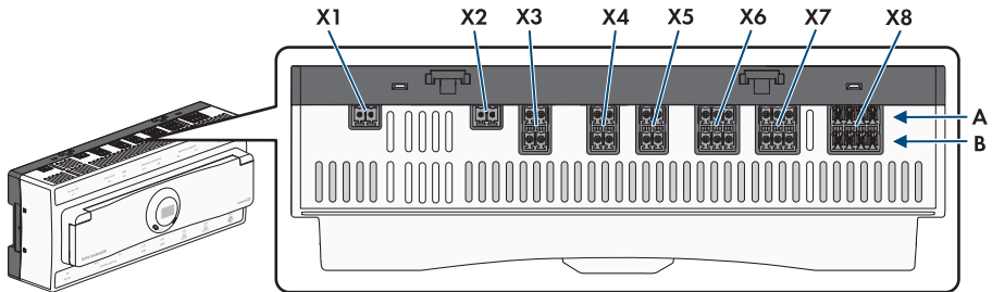
Afbeelding 6: Overzicht van bovenste aansluitpaneel
